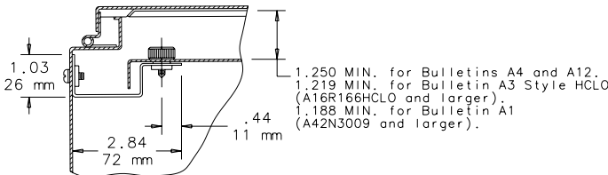
DETAIL Y
