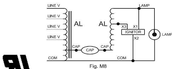
Wiring Diagram:
